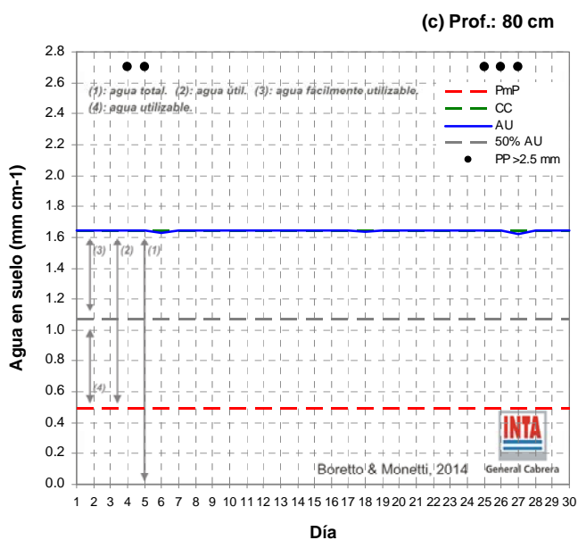
Gráfico 7a, 7b y 7c: Evolución del contenido de agua en el perfil de suelo.
