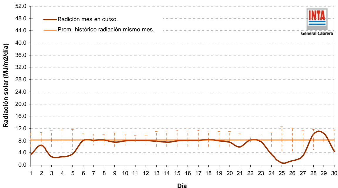
Gráfico 5: Evolución de la radiación solar del mes en curso ( serie curvilíneas ) y radiación media histórica del mismo mes ( serie rectas ) para el periodo 2001-2015. Las líneas sobre la recta histórica, representan el desvío estándar diario de la serie.
